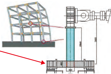
鋼構造物の部分架構試験体による柱梁接合部の耐震性能評価実験 (高速載荷試験機)
