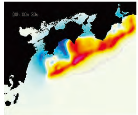
東南海・南海地震を想定した 津波波高シミュレーション
