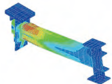
385級プレスコラムの曲げ実験・解析
